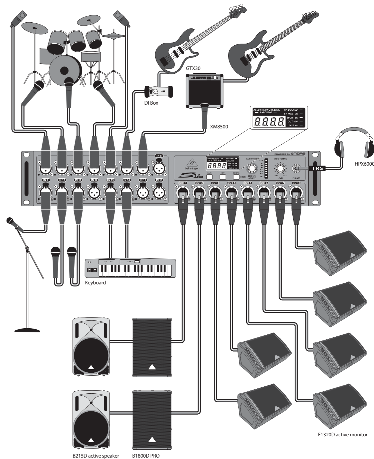
S16 フロントパネル接続例
