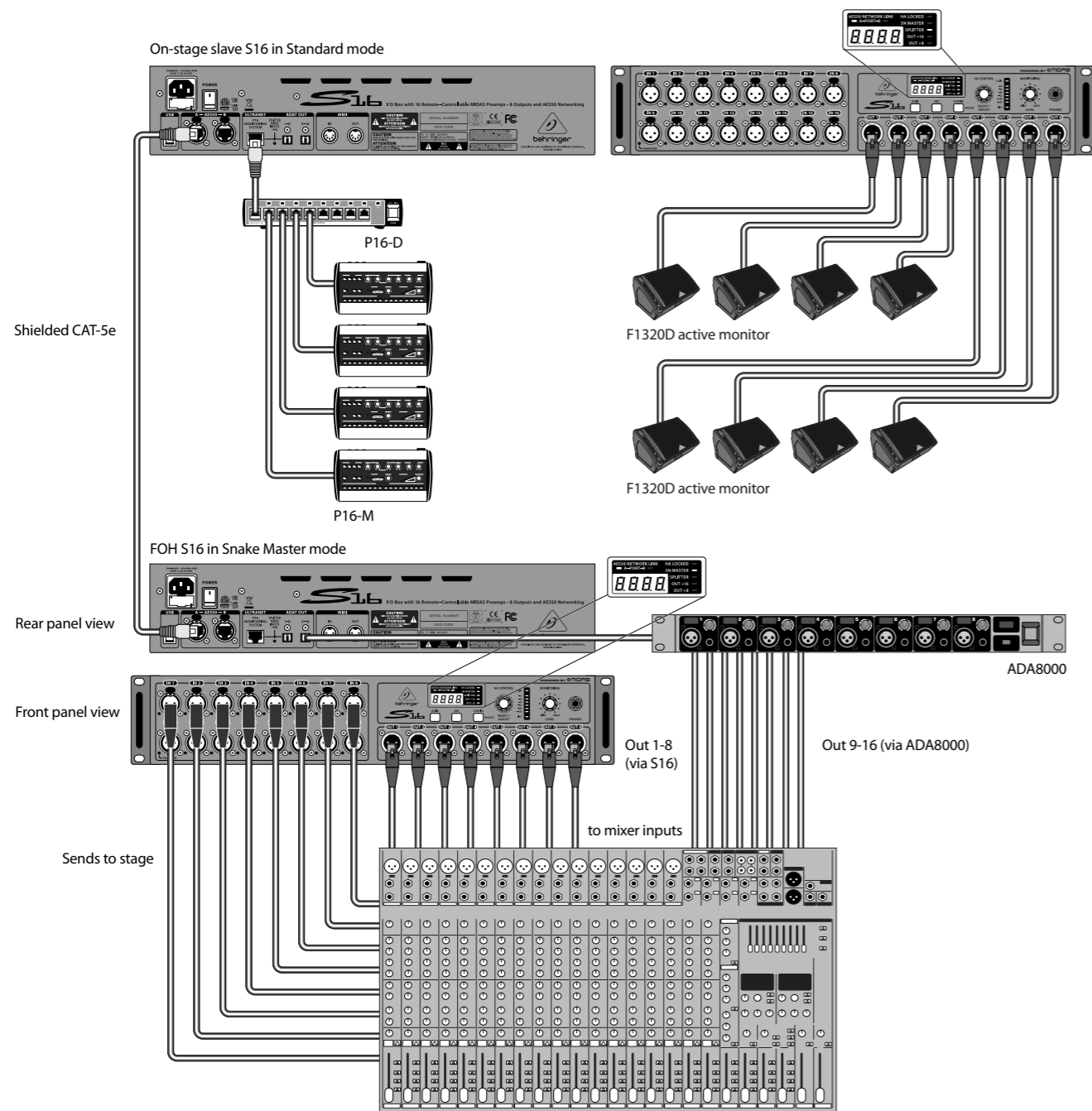
S16 スタンドアローン時接続例
